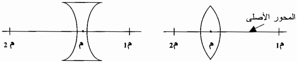
الشكل (28-2): المحور الأصلي و المركز البصري (م) ومراكز تكوير العدسة.
