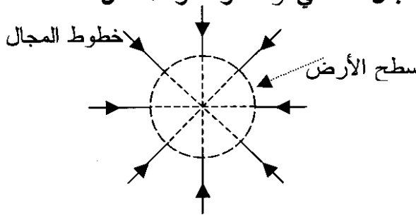
الشكل (4-1) خطوط المجال التثاقلي للأرض = خطوط قوة التثاقل
