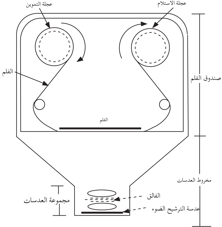
الشكل ( ١ - ٦ ) : أقسام آلة التصوير الفوتوغرافي
