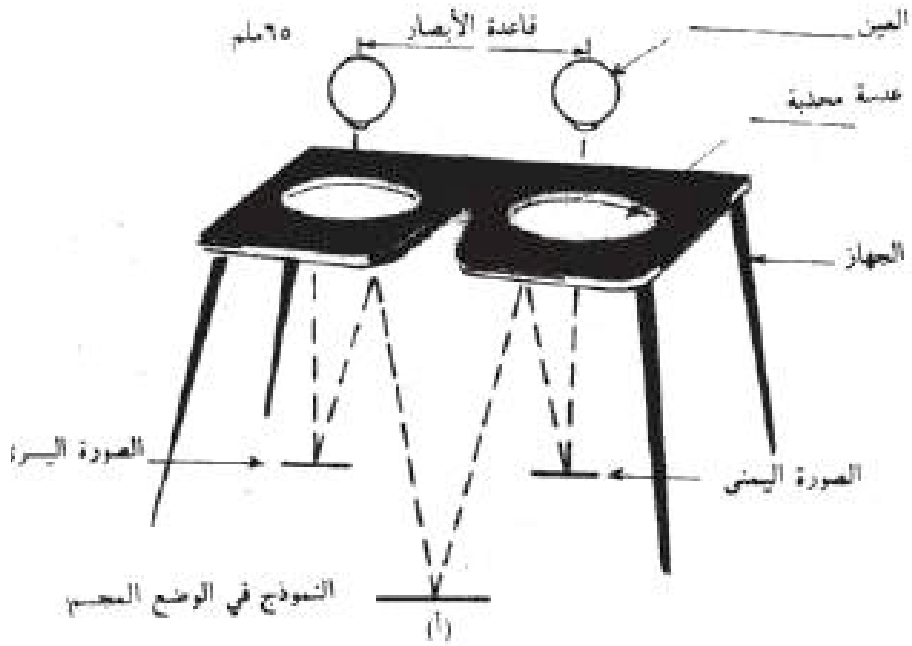
الشكل ( ١ - ٩ ) : المنظار المجسم البسيط
