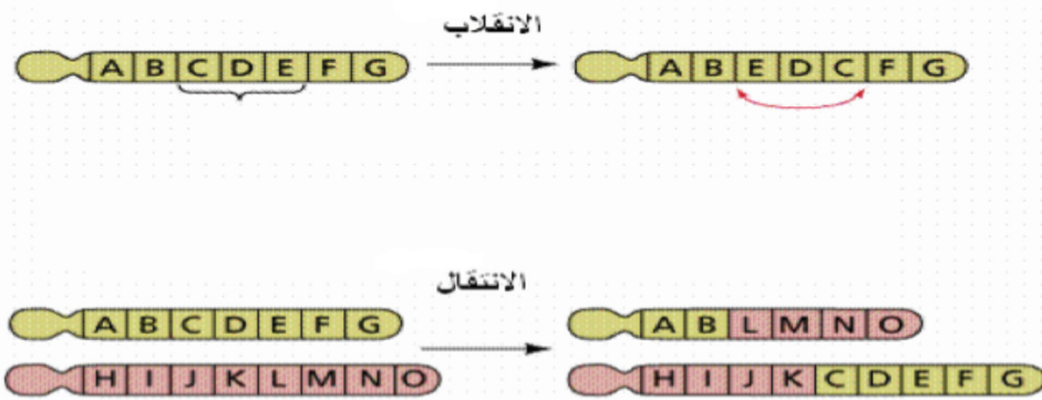
الشكل (21): الطفرات الصبغية
